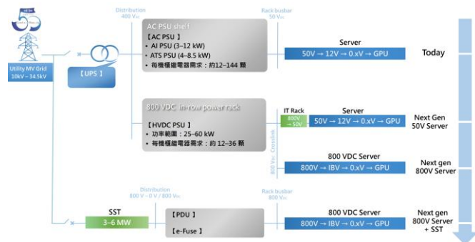
圖二、伺服器電源架構演進：AC PSU→800V HVDC→SST
